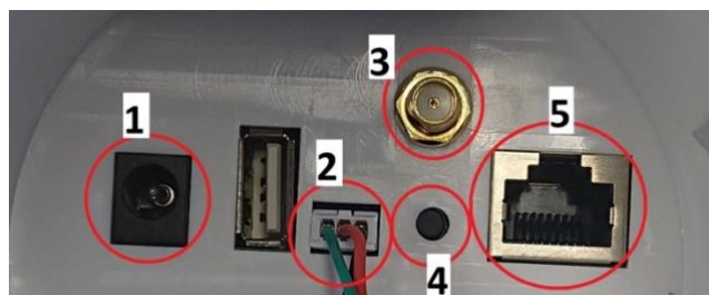
Afbeelding 2. (1) Stroombron, (2) LED connector, (3) Lora antenna connector, (4) Hard reset ( Niet gebruiken! ), (5) Ethernet poort
